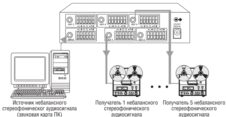
Рис. 3. Подключение VM-50AN в режиме усилителя-распределителя 1:5 небалансного стереофонического аудиосигнала
