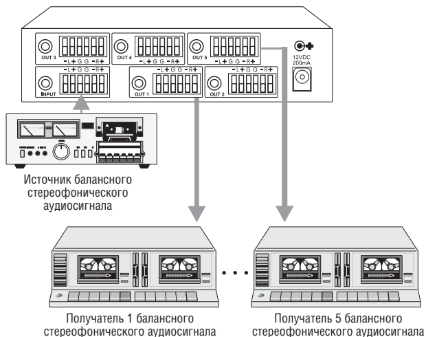
Рис. 2. Подключение VM-50AN в режиме усилителя-распределителя 1:5 балансного стереофонического аудиосигнала
