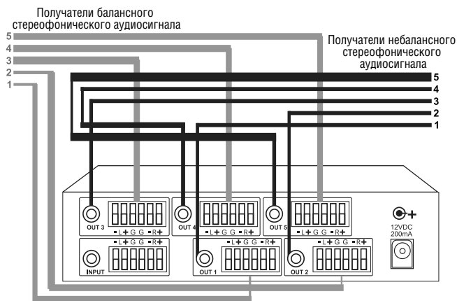
Рис. 4. Подключение VM-50AN в режиме усилителя-распределителя 1:10
