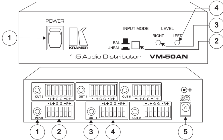
Рис. 1. Внешний вид VM-50AN
